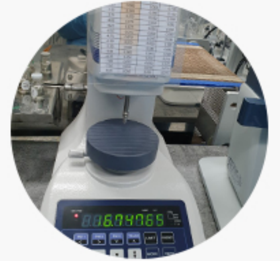
두께측정기
